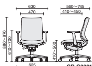
CR-G3301
