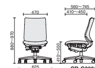
CR-G3300
